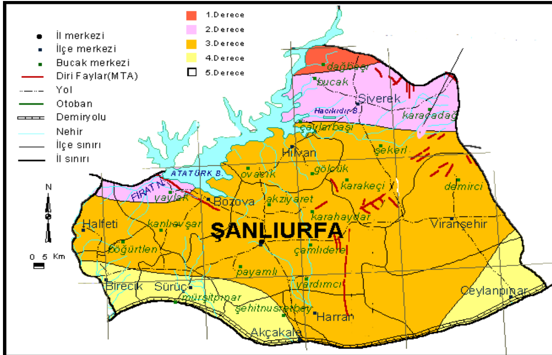
Şekil 4: Şanlıurfa İli Deprem Haritası (DAD, 1996)
