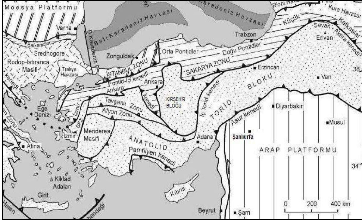
Şekil 3. Türkiye'nin Tektonik Birimleri İçerisindeki Konumu (Okay ve Tüysüz, 1999'dan)
